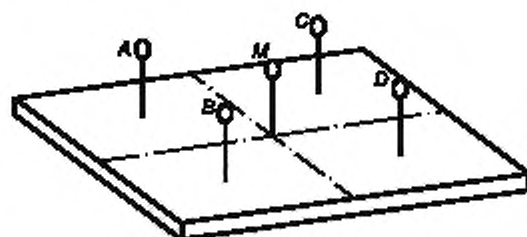
М — датчик ТЕМПЕРАТУРЫ ИНКУБАТОРА; А, В, С, D — датчики температуры воздуха.
