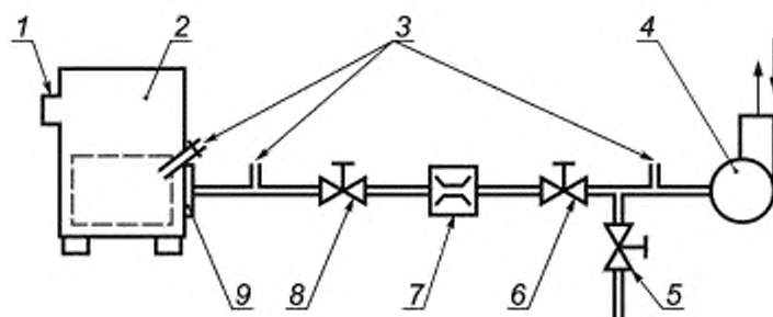
1 — выход газохода; 2 — испытуемый котел; 3 — точки измерения давления (тяги); 4 — вентилятор; 5 — клапан 3 (перепускной); 6 — клапан 2; 7 — расходомер; 8 — клапан 1 (регулирующий); 9 — горелка
