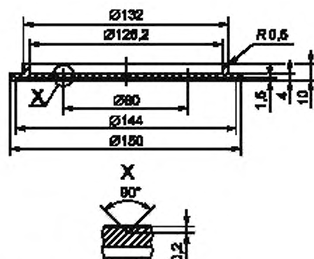
Рисунок 2 — Опорная плита
