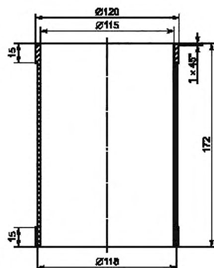
Рисунок 4 — Корпус цилиндра
