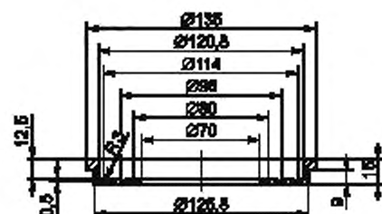
Рисунок 3 — Рамка
