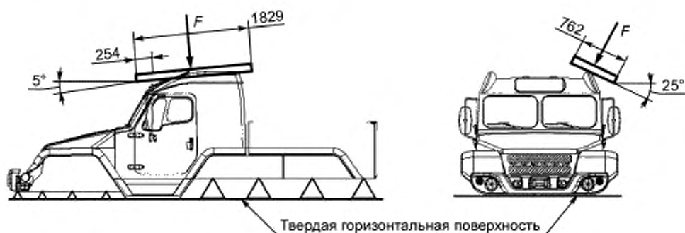
Рисунок 1 — Схема испытания защитных свойств кузова/кабины
