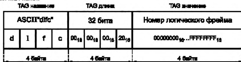
Рисунок 4 — Номер DRM логического фрейма
