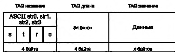
Рисунок 9 — Поток данных
