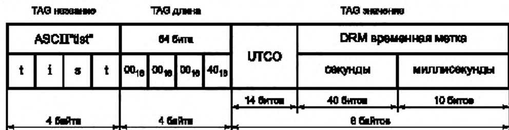
Рисунок 11 — Временная метка
