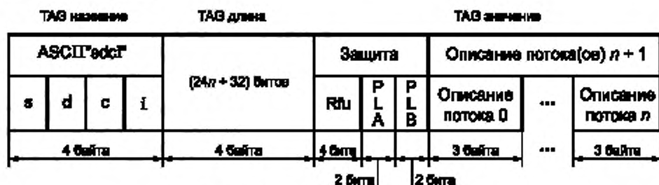
Рисунок 7 — Информация канала описания служб
