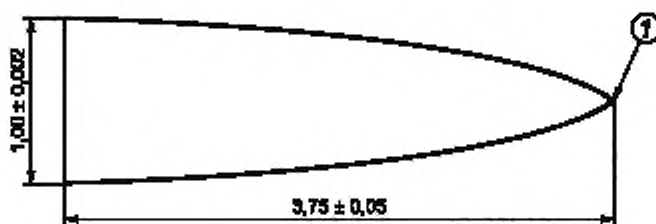
Рисунок В.1 — Игла для использования в устройстве для имитации пробоев
