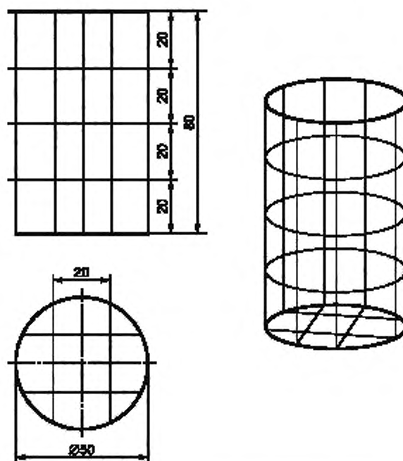
Рисунок 1 — Цилиндрическая проволочная корзина
