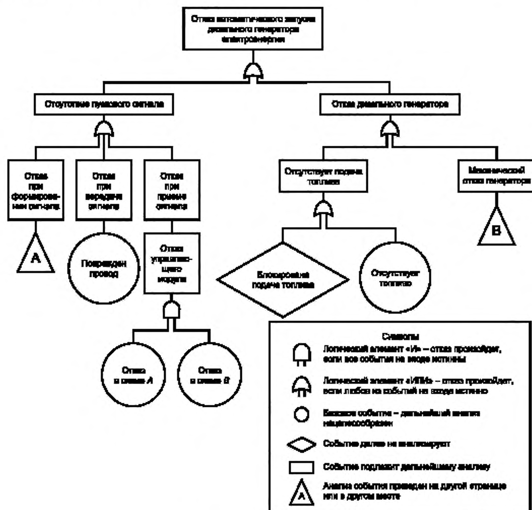
Рисунок В.2 — Пример метода FTA
