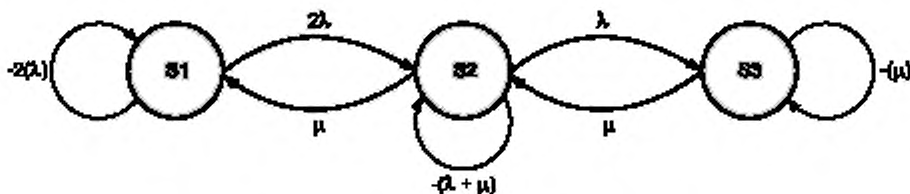
Рисунок В.10 — Пример диаграммы состояний перехода
