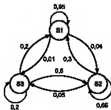
Рисунок В.9 — Пример диаграммы Маркова для системы
