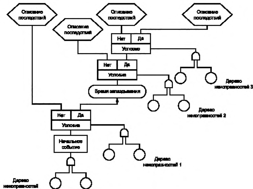
Рисунок В.4 — Пример анализа причин и последствий
