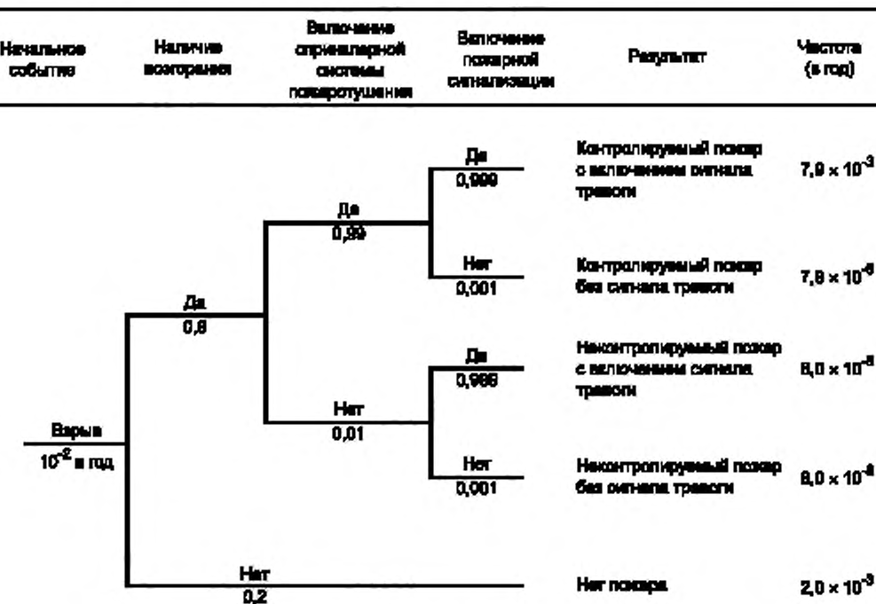
Рисунок В.3 — Пример дерева событий
