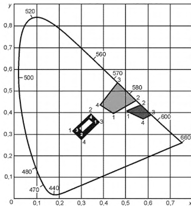
Рисунок В.1 — График цветовой области для дорожной разметки (МКО, 1931 г. [1])
