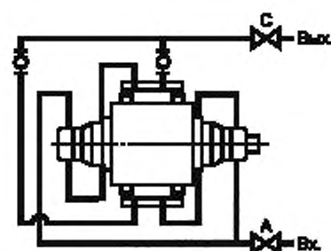
Схема Г Последовательное охлаждение опорных плит, корпуса подшипника и камеры мягкого сальника
