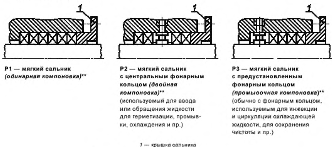
Рисунок F.1 — Примеры компоновок мягкого сальника
