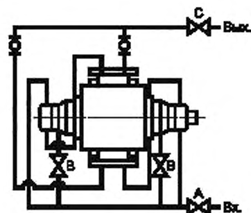
Схема Н Последовательное охлаждение опорных плит, корпуса подшипника и камеры мягкого сальника с параллельной подачей в крышку уплотнения
