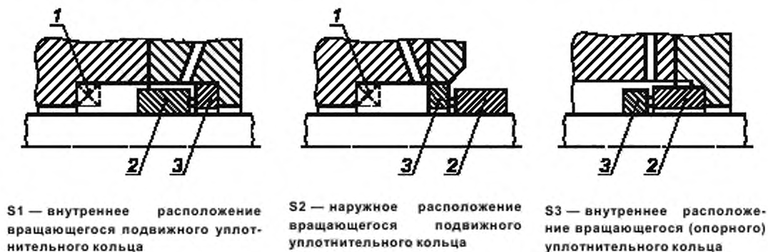
Рисунок Е.2 — Примеры компоновок одинарного торцевого уплотнения
