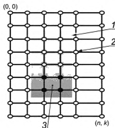
Рисунок 2 — Измерительная решетка (метод испытания В)
