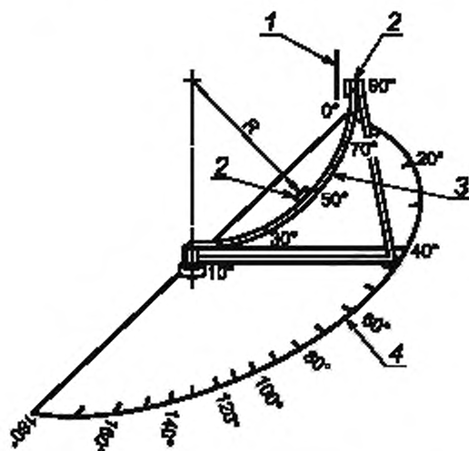
1 — съемный защитный экран; 2 — радиометр; 3 — параллель; 4 — меридиан; R — радиус, измеренный от центра окружности дуги до поверхности радиометра, величиной в пределах от 1,54 до 1,88 м. Для любого одного измерения радиус дуги не должен изменяться больше чем на \pm 20 мм
