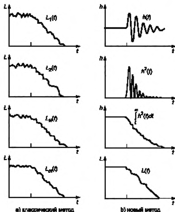
L — уровень звукового давления; h — импульсная переходная характеристика; t — время
