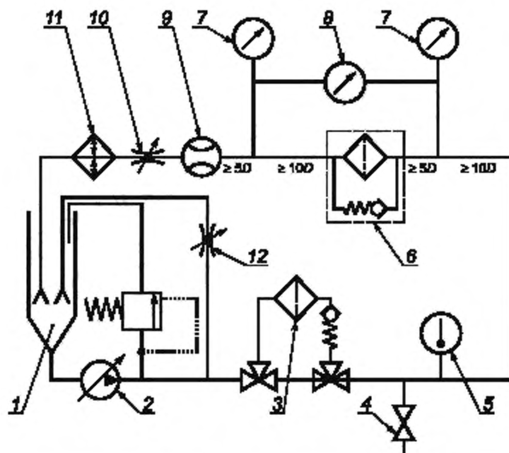
1 — гидробак; 2 — насос с регулируемым потоком; 3 — фильтр предварительной очистки; 4 — клапан для отбора проб; 5 — термометр; 6 — испытуемый фильтр с перепускным клапаном; 7 — датчик абсолютного давления; 8 — датчик дифференциального давления; 9 — расходомер; 10 — дроссель; 11 — теплообменник; 12 — дроссель для регулировки расхода
