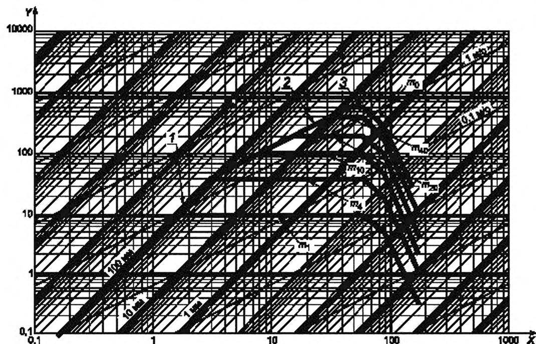
X — частота, Гц, Y — ускорение, м/с 2 ; 1 — предел по перемещению; 2 — предел по скорости; 3 — максимальное ускорение
