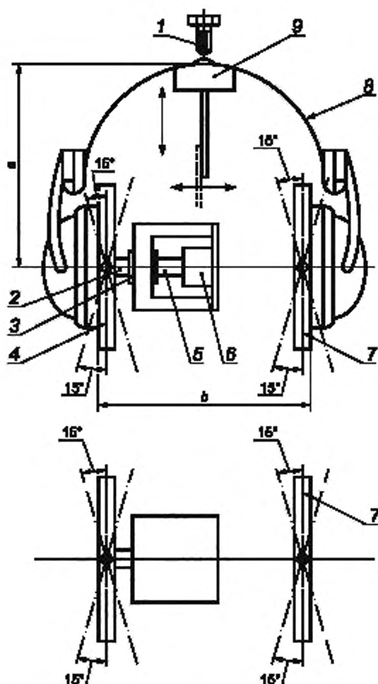
1 — монтажный болт; 2 — ось; 3 — линейный подшипник; 4 — опорная пластина; 5 — соединительный штифт; 6 — датчик силы; 7 — регулируемая пластина; 8 — корпус каски со снятым мягким креплением; 9 — опорная площадка для каски сферическим радиусом 95 мм; a — тестовая высота, b — тестовая ширина
