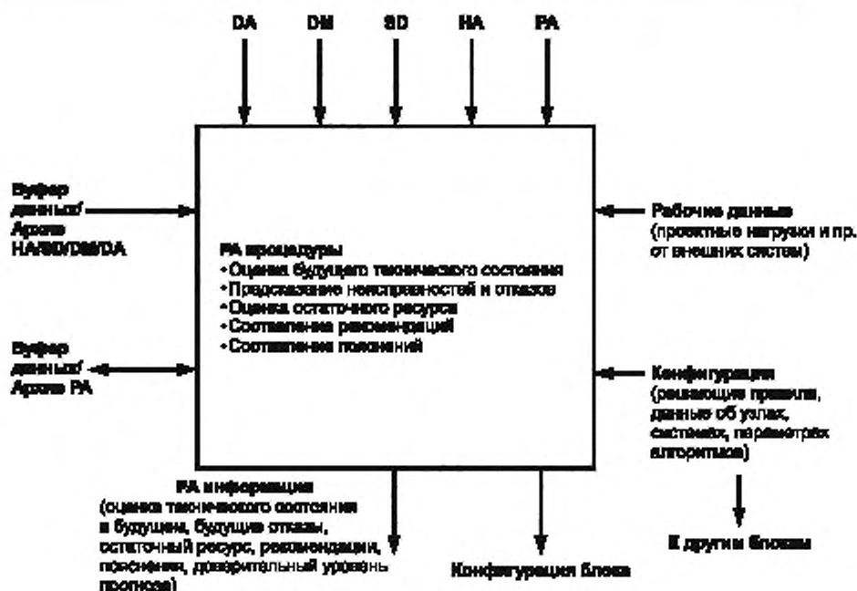
Рисунок 7 — Блок составления прогноза
