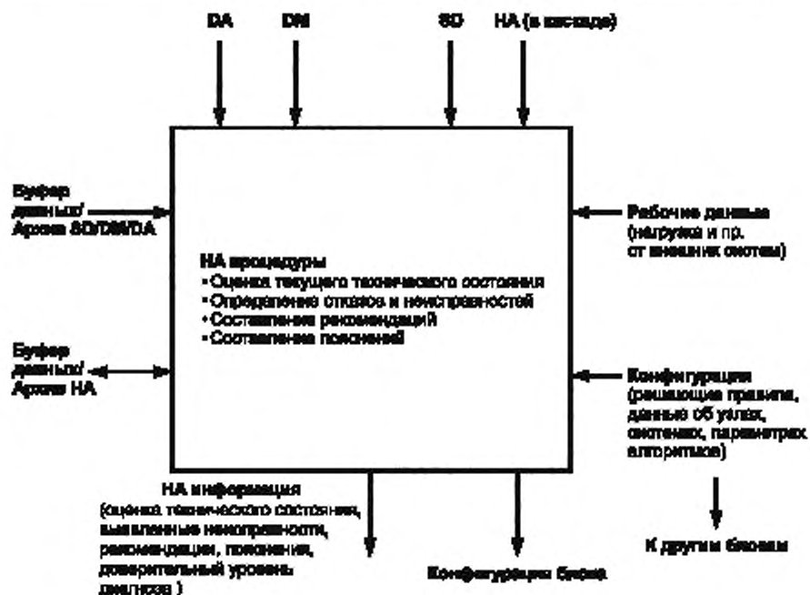
Рисунок 6 — Блок составления диагноза
