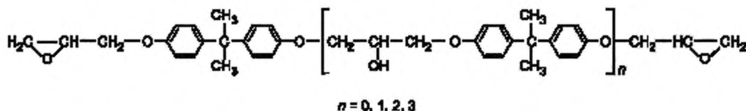
Рисунок А.1 — Молекулярная структура эпоксидной смолы
