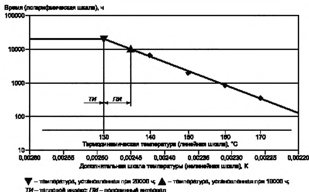
Рисунок А.2 — График теплостойкости
