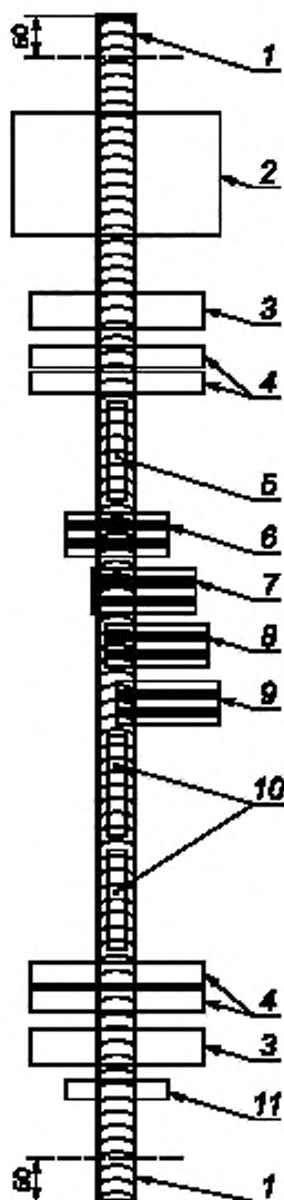
Рисунок С.1 — Отбор образцов для испытаний из продольных сварных швов, изготовленных труб или трубных деталей для проведения аттестации технологии сварки
