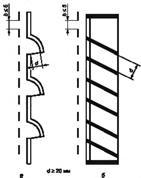
Рисунок А.23 — Вентиляционные отверстия для непищевой зоны
