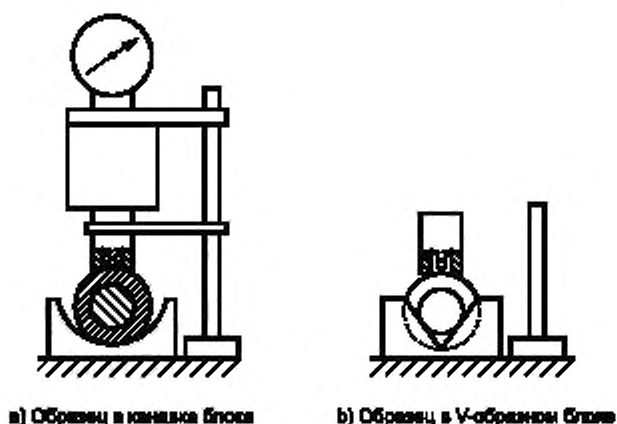
Рисунок Е.2 — Испытание на поверхности с небольшим радиусом кривизны
