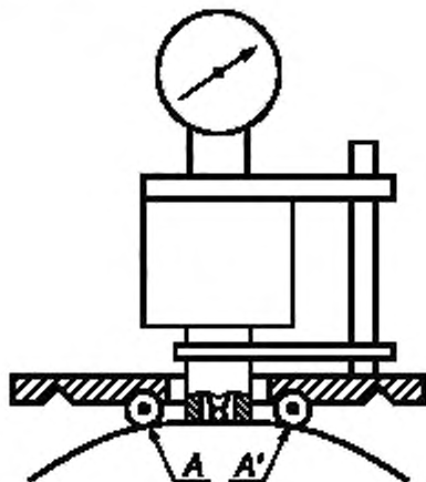
Рисунок Е.1 — Испытание на поверхности с большим радиусом кривизны
