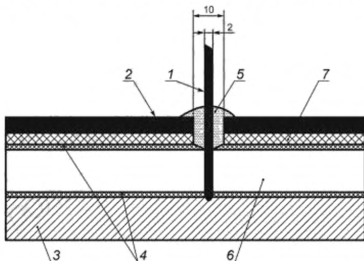
Рисунок А.2 — Расположение термопар на токопроводящей жиле стандартного контура
