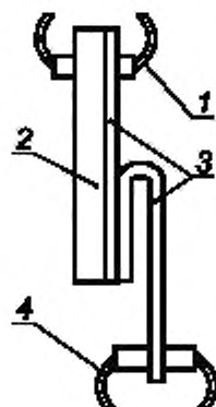
Рисунок G.3 — Прочность отслаивания металлической ленты, наложенной с перекрытием
