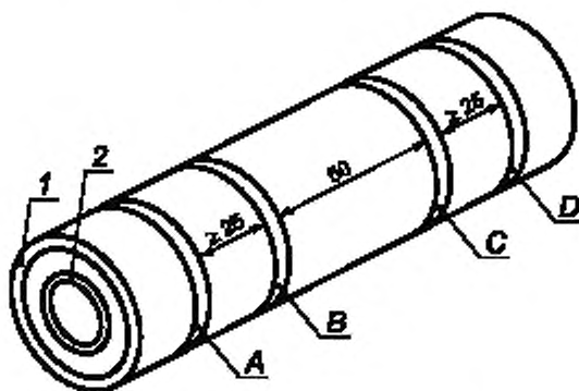
1 — экран по изоляции; 2 — экран по жиле; A, D — электроды тока; B, C — электроды напряжения
