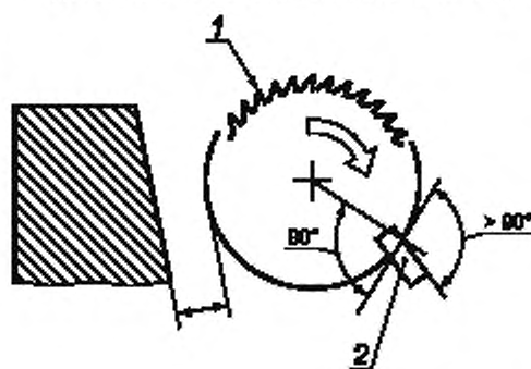
1 — зубчатый барабан; 2 — очищающая гребенка
