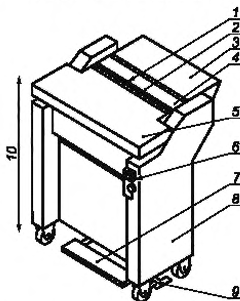
1 — зубчатый барабан; 2 — нож; 3 — стол разгрузки; 4 — держатель ножа; 5 — стол подачи; 6 — выключатель ON/OFF; 7 — ножной выключатель; 8 — двигатель; 9 — блокировочное устройство; 10 — высота стола
