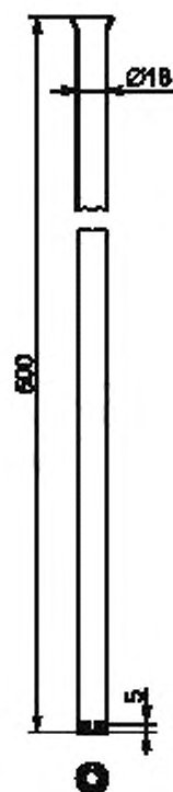
Рисунок А.2 — Трубка, вставляемая в пробирку
