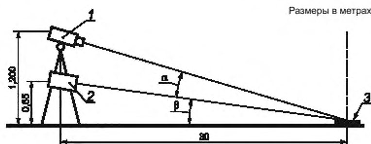
1 — фотоприемник; 2 — стандартный прожекторный источник света типа А по ГОСТ 7721; 3 — дорожная разметка
