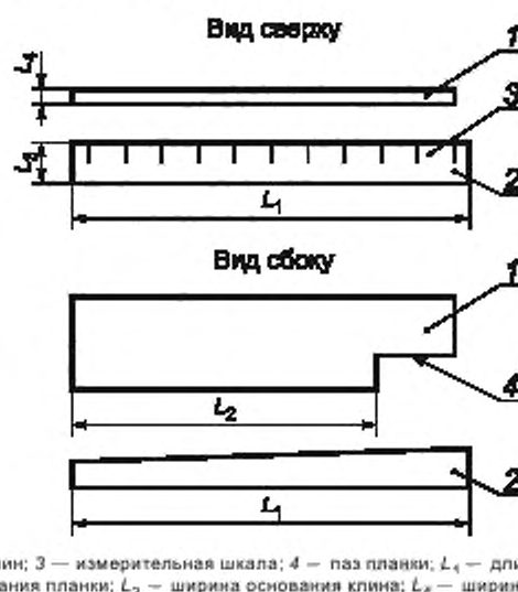
Рисунок 1 — Схема высотомера для определения высоты выступания горизонтальной дорожной разметки над поверхностью, на которую она нанесена
