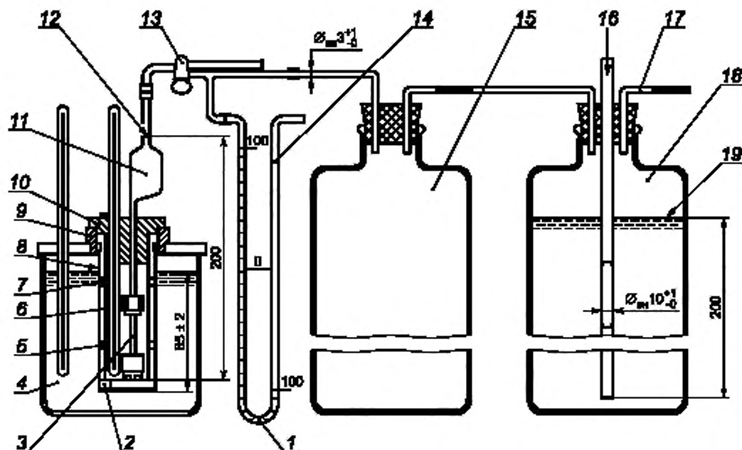
1 — вода; 2 — изолирующее кольцо; 3 — фильтр; 4 — охлаждающая баня; 5, 7 — прокладка; 6 — испытательный сосуд; 8 — кожух; 9 — поддерживающее кольцо; 10 — пробка; 11 — пилетка; 12 — отметка 20 см 3 ; 13 — запорный кран с двойным наклонным каналом; 14 — U-образный манометр; 15 — дополнительный вакуумный резервуар; 16 — воздушный клапан; 17 — источник вакуума; 18 — вакуумный резервуар; 19 — уровень воды
