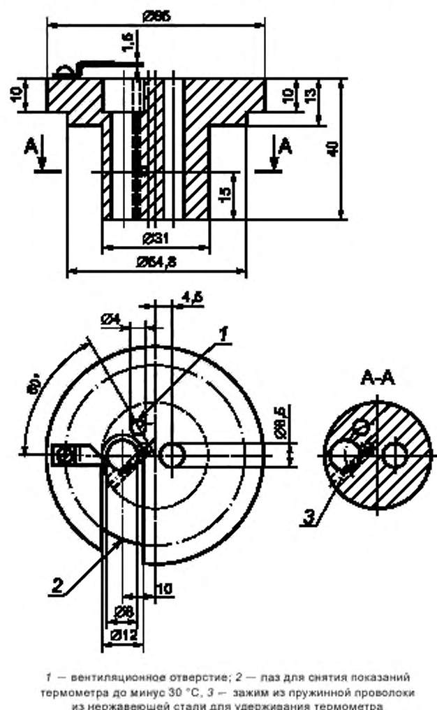
Рисунок 5 — Пробка с отверстиями для пипетки, термометра и вентиляции
