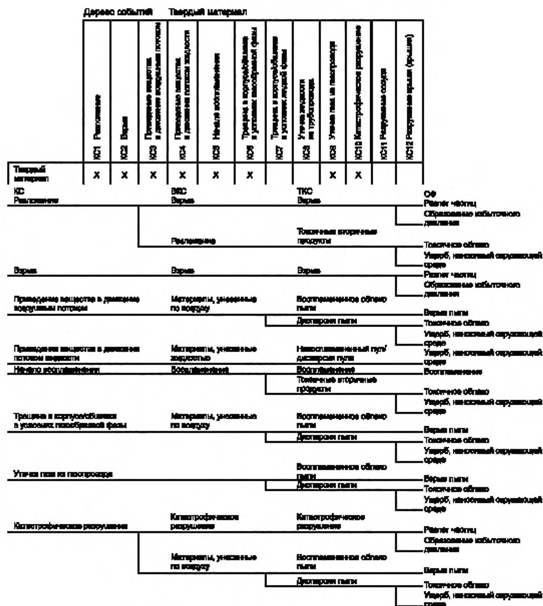
Рисунок А.1 — Дерево событий для твердых материалов
