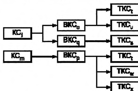
Рисунок 4 — Пример построения дерева событий (до ТКС)
