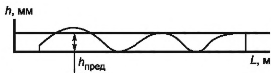
Рисунок 10.3 — График зависимости параметра h от длины пути L
