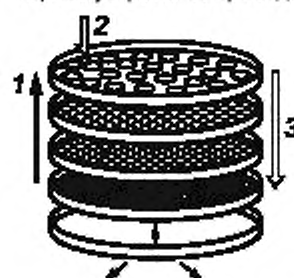
1 — направление увеличения диаметра отверстий; 2 — загрузка материала; 3 — направление движения материала
