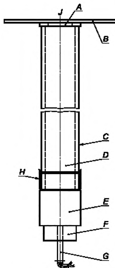
A — прокладки; B — контрольная пластина, C — стальная труба; D — испытуемая химическая продукция; E — бустер, состоящий из циклотриметилентринитрамина/парафина или ТЭН/тринила; F — держатель детонатора; G — детонатор, H — пластмассовая мембрана, J — датчик скорости
