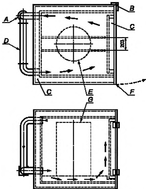
А — вентилятор; В — шарниры; С — изоляция; D — нагреватель; Е — барабан; F — зазор; G — барабан (например, 0,58 × 0,89 м)
