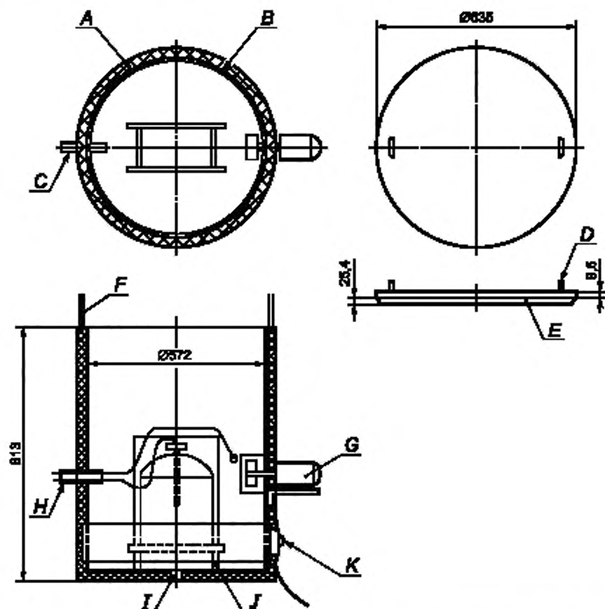
А — изоляция толщиной 25 мм; В — барабан без днища, 220 л; С — труба, 19 мм; D — стержень с петлей, 9,6 мм; E — изоляция на стальном покрытии; F — контрольный кабель, 3 мм; G — вентилятор; H — термпары и контрольные приборы, I — дренаж, J — угловая стойка, 25 мм, K — нагреватель барабана, 2 кВт
