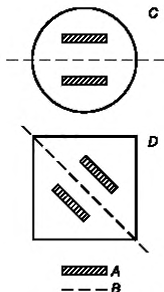
А — заряды взрывчатой химической продукции; В — линия симметрии; С — цилиндрическая упаковка (вид сверху). D — прямоугольная упаковка (вид сверху)
