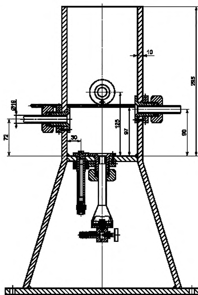
Рисунок 10 — Защитно-нагревательное устройство
