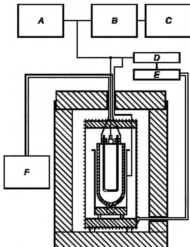
A — многооточный регистратор и регулятор температуры (10 мВ); B — наружная установка на ноль; C — записывающее устройство высокой точности; D — управление, E — реле; F — внутренний первичный нагреватель
