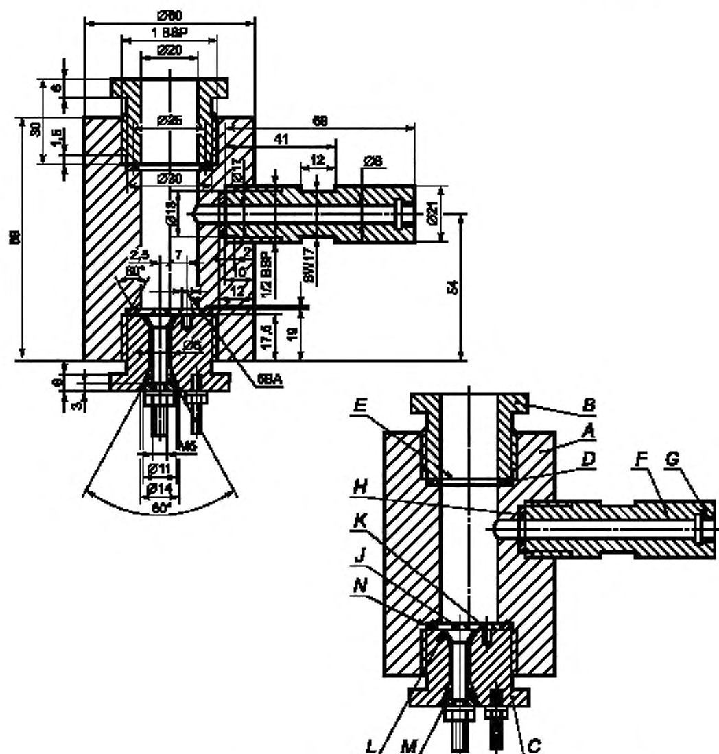
А — корпус сосуда высокого давления; В — фиксирующая пробка разрывной мембраны; С — запальная пробка; D — мягкая свинцовая прокладка; E — разрывная мембрана; F — боковое ответвление; G — резьба датчика давления; H — медная прокладка; J — изолированный электрод; K — заземленный электрод; L — изоляция; M — стальной конус; N — паз смещения прокладки
