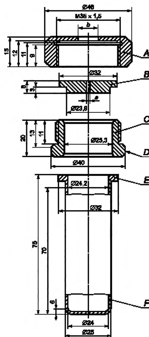
А — гайка ( b = 10,0 или 20,0 мм), рассчитанная на гаечный ключ 41; В — пластина с отверстием ( a = 1,0 \times 20,0 мм в диаметре); С — резьбовое кольцо; D — фаски для гаечного ключа 36; E — фланец; F — трубка
