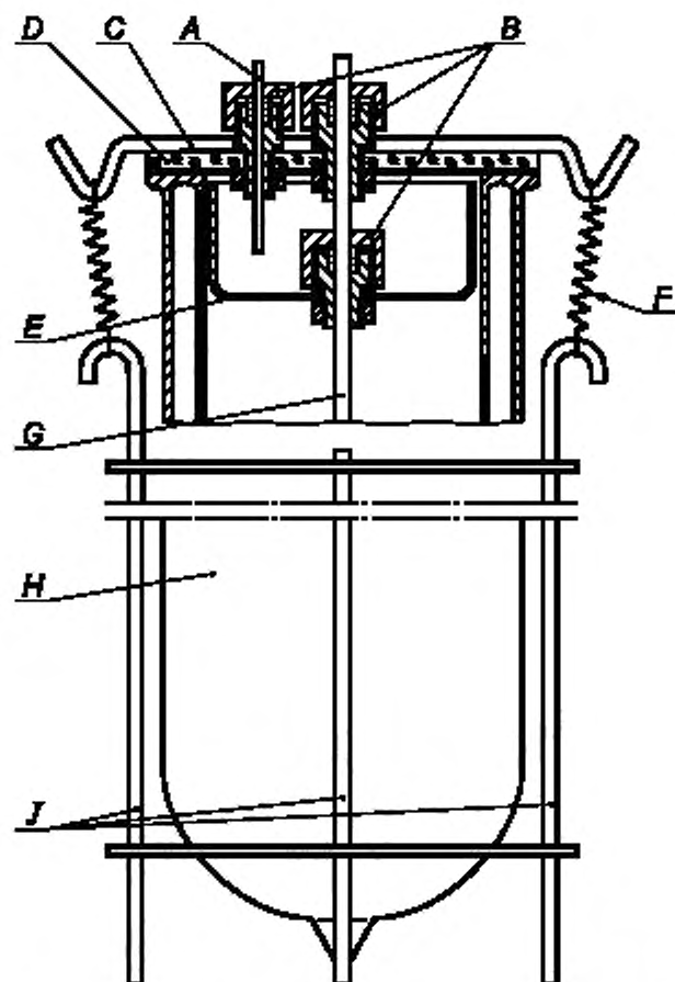
А — капиллярная трубка из ПТФЭ; В — специальные заворачивающиеся заглушки (из ПТФЭ или алюминия) с уплотнительными кольцами; С — металлическая планка; D — стеклянная крышка; E — основание стеклянного резервуара; F — пружина; G — стеклянная защитная трубка; H — сосуд Дьюара; J — стальное поддерживающее устройство
