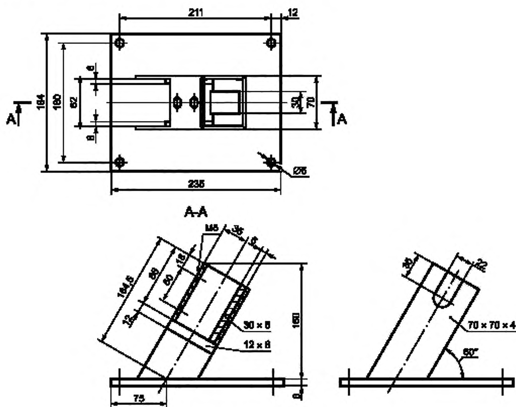
Рисунок 5 — Опорный стенд
