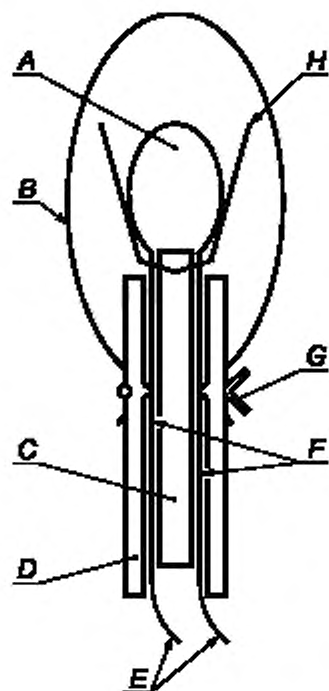
А — мостик накалывания; В — пленка из поливинилхлорида; С — изоляция; D — трубка из кремнийорганического каучука; Е — запальные выводы; F — контакты из фольги; G — проволока для водонепроницаемой герметизации; H — запальный кембрик
