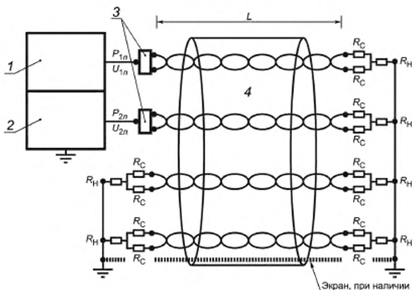
1 — анализатор цепей или генератор сигналов; 2 — анализатор цепей или измерительный приемник; 3 — симметрирующий трансформатор; 4 — измеряемый кабель; R_C и R_H — нагрузки симметричной и несимметричной цепей соответственно. P_{1n}(U_{1n}) — мощность (напряжение) сигнала на ближнем конце подверженной влиянию пары; P_{2n}(U_{2n}) — мощность (напряжение) сигнала на ближнем конце подверженной влиянию пары
