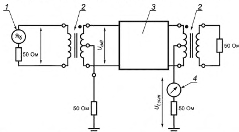
Рисунок 7 — Схема измерения затухания асимметрии на ближнем конце
