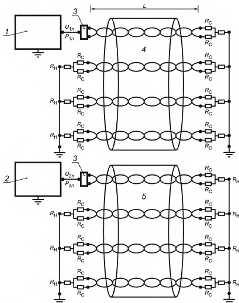
1 — анализатор цепей или генератор сигналов, 2 — анализатор цепей или измерительный приемник; 3 — симметрирующий трансформатор; 4 — влияющий кабель, 5 — подверженный влиянию кабель; R_C и R_n — нагрузка симметричной и несимметричной цепей соответственно; L — длина измеряемых кабелей; P_{1n}(U_{1n}) — мощность (напряжение) сигнала на ближнем конце влияющей пары влияющего кабеля; P_{2n}(U_{2n}) — мощность (напряжение) сигнала на ближнем конце подверженной влиянию пары подверженного влиянию кабеля
