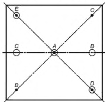
Рисунок Д.4 — Расположение термопар на рабочих поверхностях плит нагревателя и холодильника
