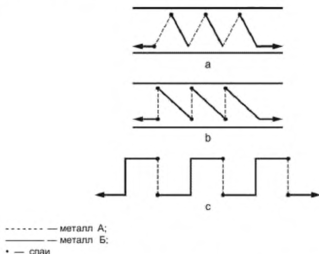
Рисунок D.7 — Примеры расположения спаев термопар термобатарей
