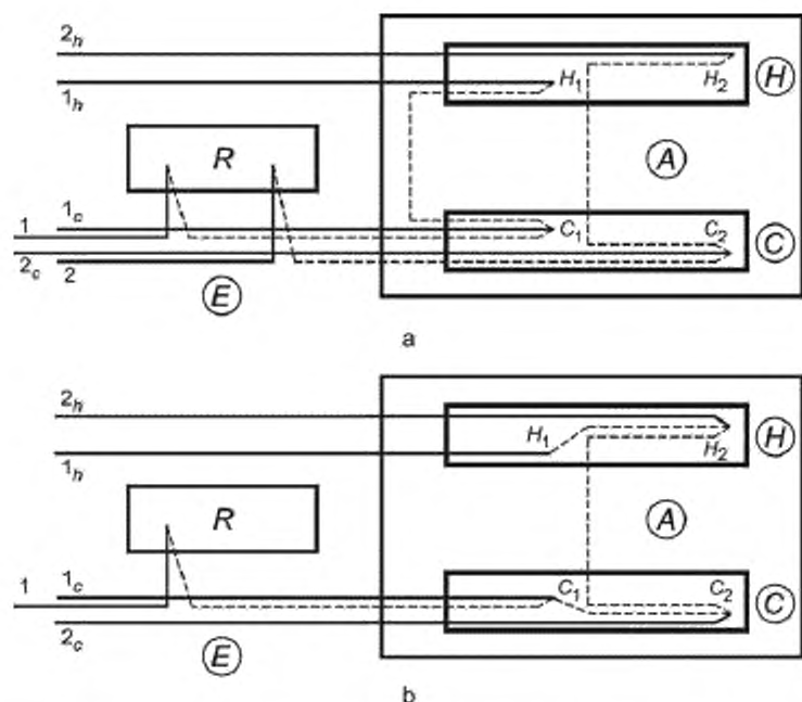
H — нагреватель; H_1, H_2 — спай термопар, установленных на нагревателе; C — холодильник; C_1, C_2 — спай термопар, установленных на холодильнике; R — эталонный термостат (точка плавления льда); A — корпус прибора; E — окружающая среда (лаборатория)
