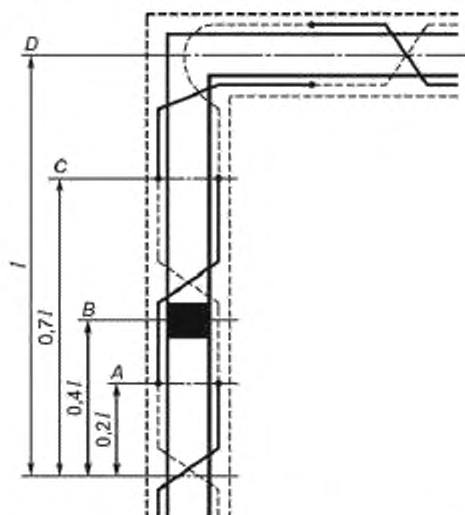
Рисунок Д.2 — Расположение слейсера (прокладки) и слаяв проводов уравнивающей термобатареи
