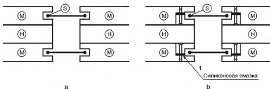
Рисунок Д.2 — Расположение слейсера (прокладки) и слаяв проводов уравнивающей термобатареи
