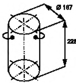
Рисунок 2 — Малый контейнер
