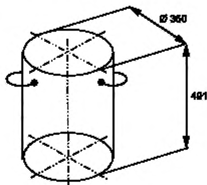
Рисунок 1 — Большой контейнер
