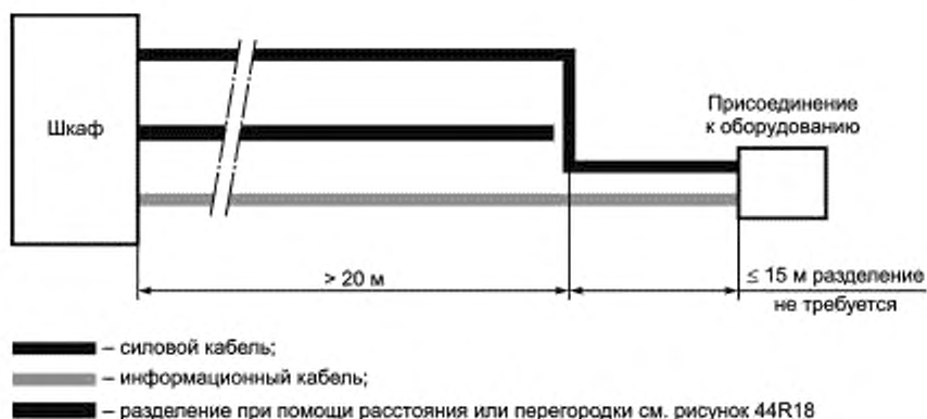
Рисунок 44.R17B — Разделение силовых и информационных кабелей при длинах кабельной трассы > 35 \text{ м}
