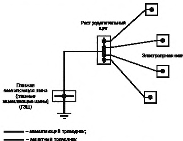
Рисунок 44.R13 — Примеры радиального соединения защитных проводников
