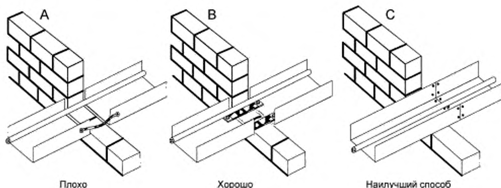
Рисунок 44.R 22 — Соединение металлических секций
