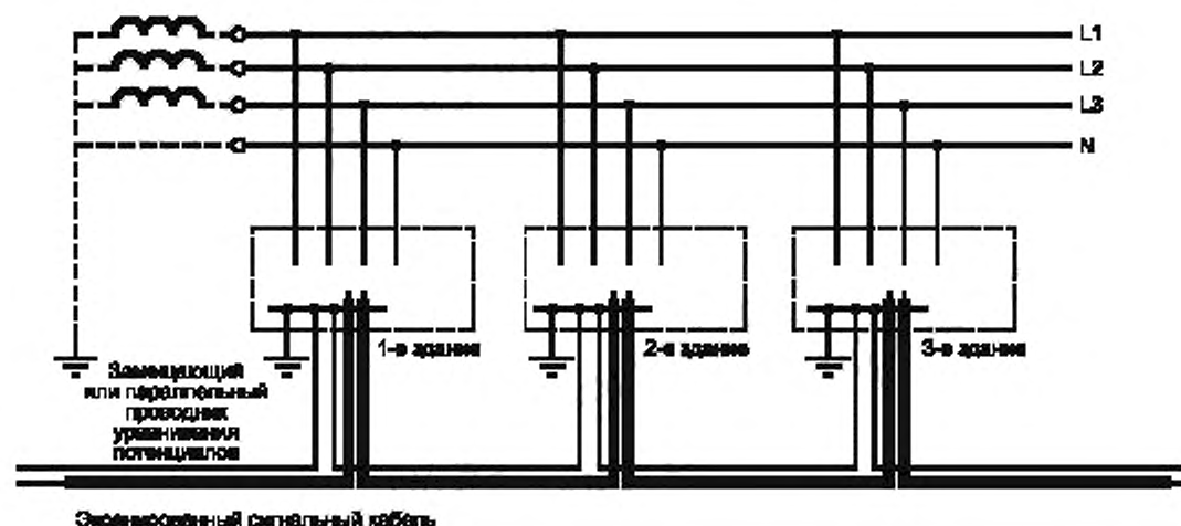
Рисунок 44.R2 — Пример заземляющего или шунтирующего проводника уравнивания потенциалов в системе ТТ
