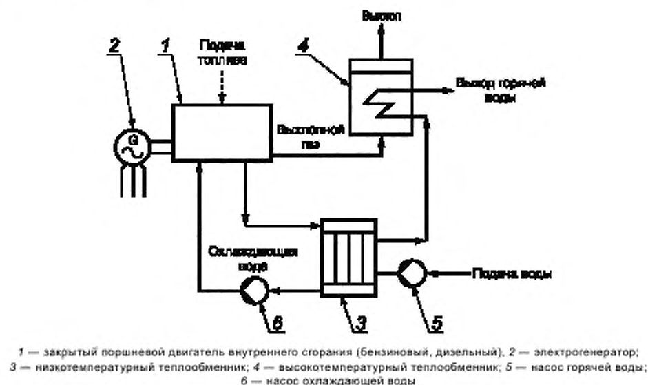
Рисунок С.3 — Типовая схема КГУ с поршневым двигателем внутреннего сгорания (поршневой ДВС — КГУ с горячей водой)
