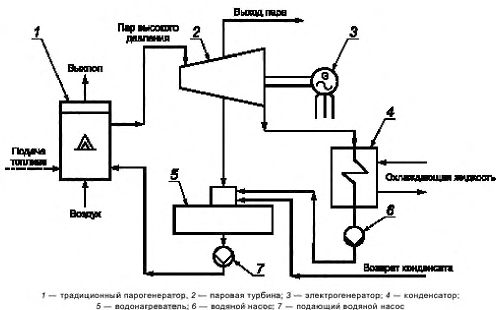
Рисунок С.4 — Типовая схема КГУ с паровой турбиной (конденсационная паровая турбина с технологическим паром)
