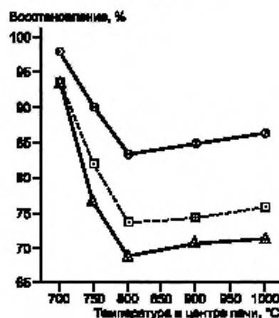
Система окисления серы: тиофен в циклогексане (10 ppm в) с использованием электролита с концентрацией анида, равной 0,00 %
