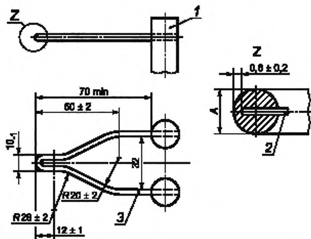
1 — щиты; 2 — термопара; 3 — раскаленная проволока
