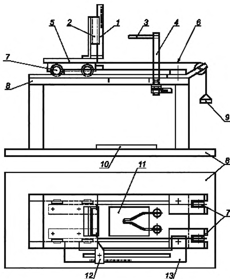
1 — шкала для измерения высоты пламени; 2 — опора для испытуемого образца (см. рисунок 4); 3 — раскаленная проволока, 4 — штырь — держатель раскаленной проволоки; 5 — тележка, 6 — натяжной шнур, 7 — ролики с низким коэффициентом трения; 8 — плита основания, 9 — груз, 10 — специальный слой; 11 — отверстие в плите основания для падающих частиц; 12 — регулируемый упор; 13 — регулятор проникновения
