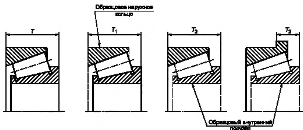
T — ширина (монтажная высота) роликового конического подшипника; T_1 — монтажная высота внутреннего поддула роликового конического подшипника; T_2 — монтажная высота наружного кольца роликового конического подшипника
