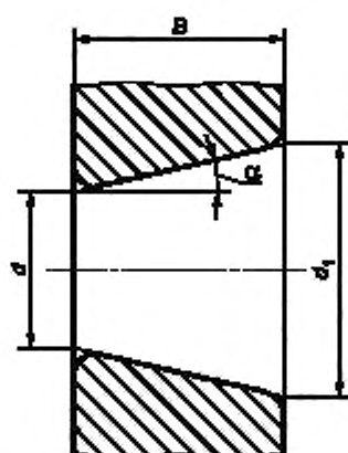
Рисунок 4 — Номинальное коническое отверстие
