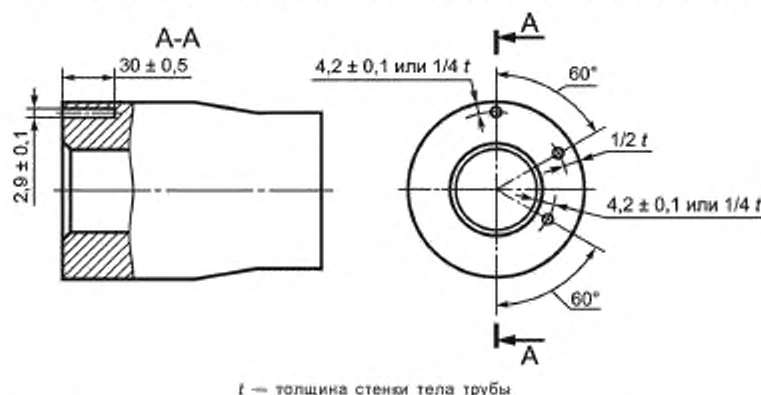
а — Стандартный образец с искусственным дефектом типа «радиальное сверленное отверстие»
