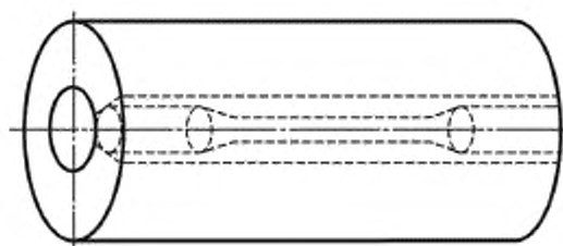
b — Цилиндрический образец для испытания на растяжение
