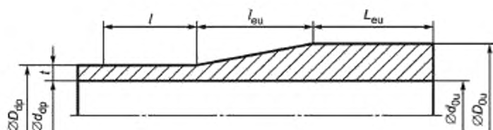
б — Наружная высадка, группы прочности D и E (все размеры, кроме бурильных труб наружным диаметром тела трубы 88,90 мм и толщиной стенки трубы 9,35 мм. имеющих незначительную внутреннюю высадку)
