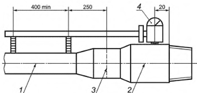
д -- Измерение соосности тела бурильной трубы и замка
