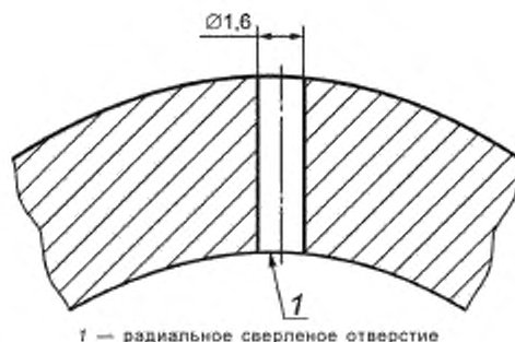
а — Стандартный образец с искусственным дефектом типа «радиальное сверленное отверстие»
