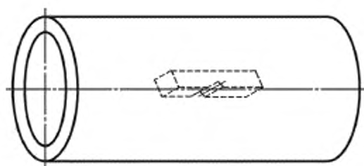
a — Образец для испытания на ударный изгиб
