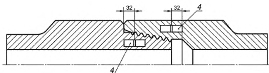
с — Расположение образцов для испытания на ударный изгиб для ниппеля и муфты
