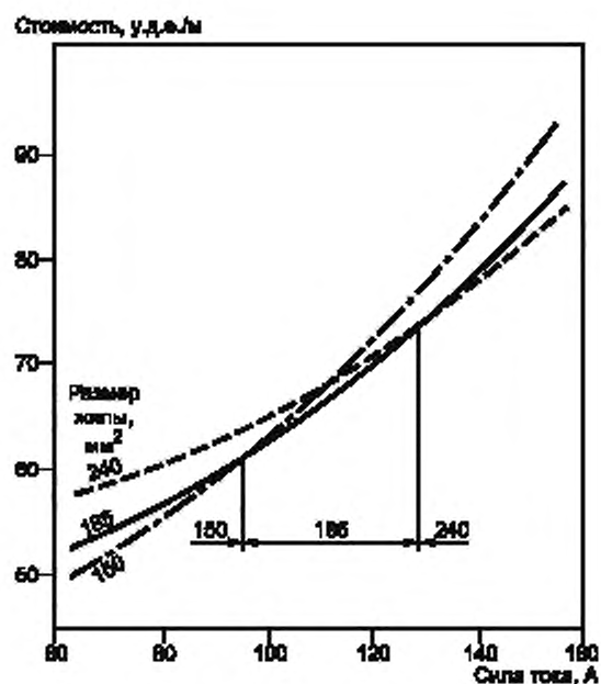
Рисунок А.2 — Диапазоны экономичных токов
