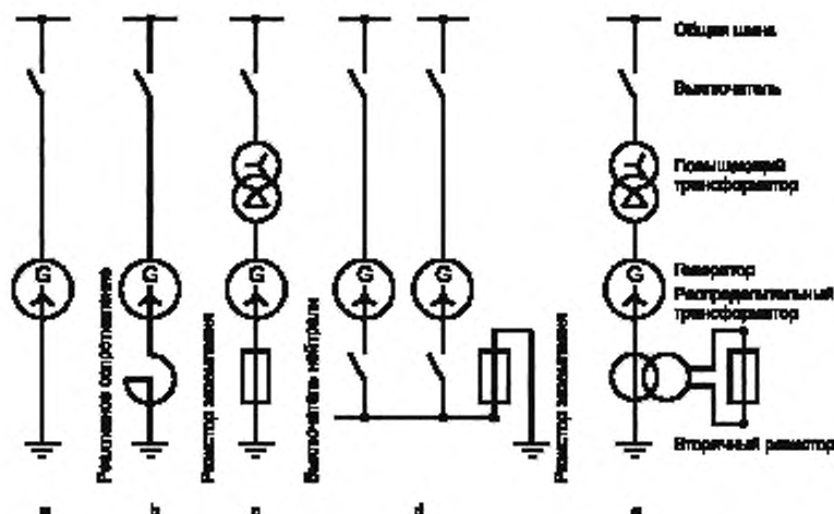
Типы заземления нейтрали: а — глухое заземление; б — заземление через реактивное сопротивление; в — заземление низкого сопротивления; г — заземление низкого сопротивления системы с несколькими источниками (один заземляющий резистор и коммутационное устройство); д — заземление низкого сопротивления системы с несколькими источниками (один заземляющий резистор и коммутационное устройство); е — распределительный трансформатор (заземление в вторичном резисторе); G — генератор
