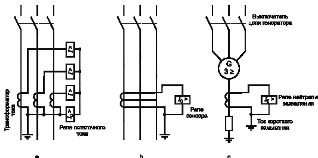
Рисунок 3 — Защита от короткого замыкания на землю с обнаружением тока нулевой последовательности
