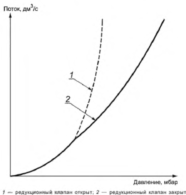
Рисунок 8 — Характеристика потока (13.3.10)
