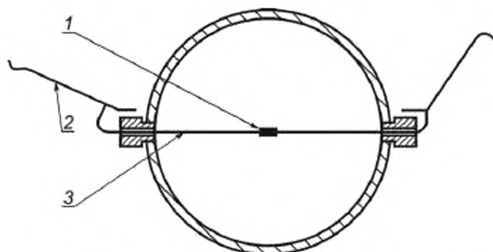
Рисунок 3 — Установка термопары (11.6.1.1)
