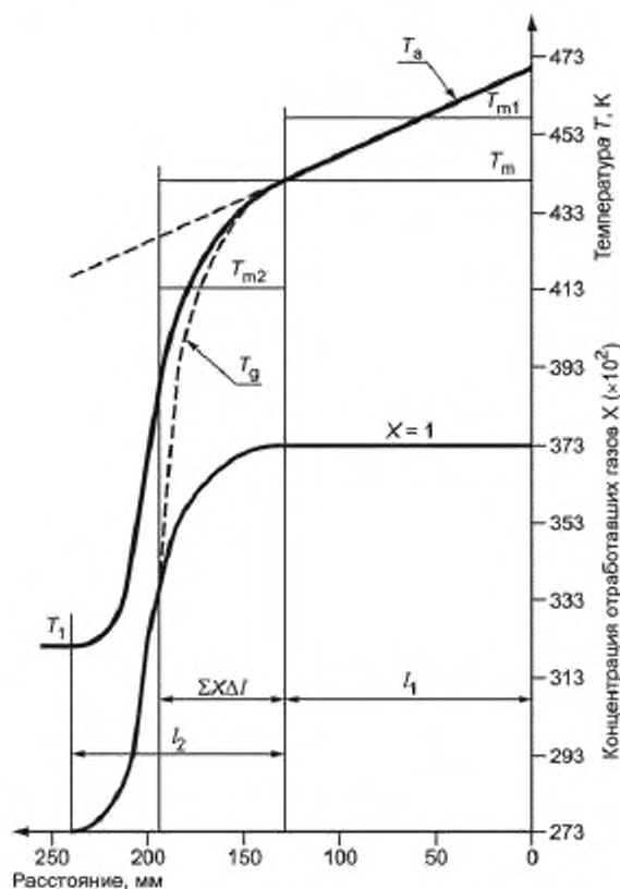
Рисунок А.2 — Практический пример использования описанного метода
