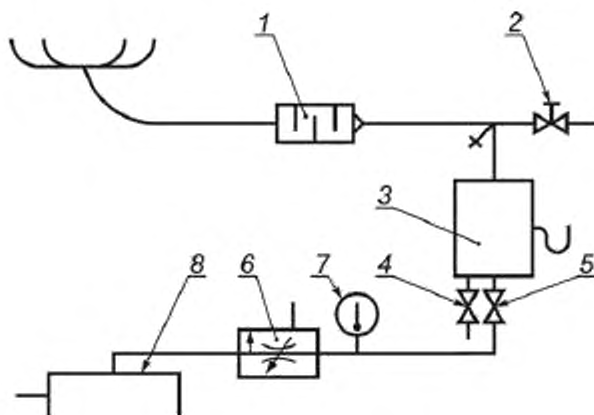
Рисунок 4 — Дымомер с источником света от лампы накаливания (11.6.3)
