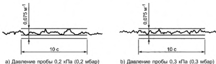
Рисунок 7 — Неустойчивость значений (13.3.2.2)
