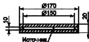
Рисунок 1 — Кювета
