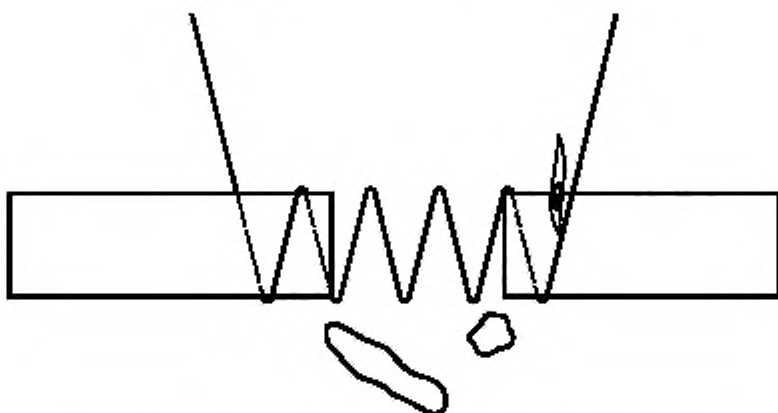
Рисунок С.5 — Воспламенение с частичным сквозным проплаванием. Результат испытания — воспламенение есть
