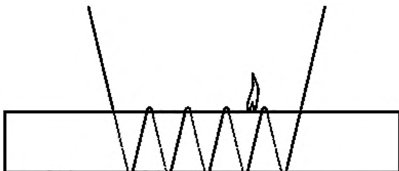
Рисунок С.4 — Воспламенение без сквозного проплавания. Результат испытания — воспламенение есть
