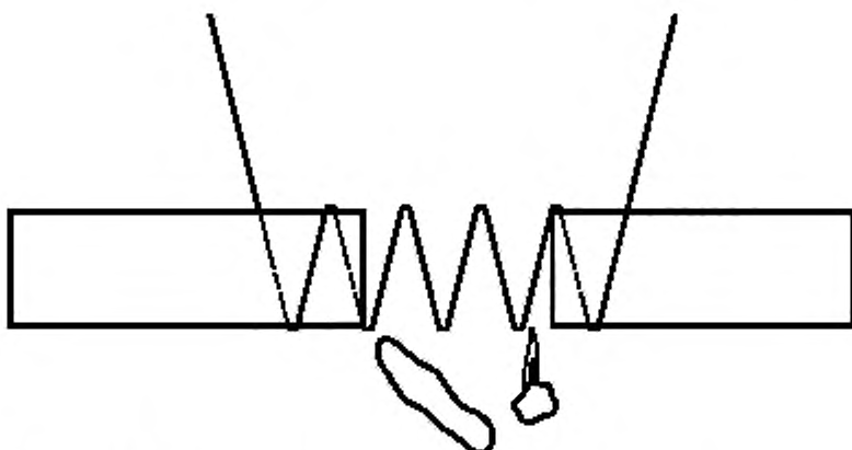
Рисунок С.6 — Воспламенение с частичным или полным сквозным проплаванием. Результат испытания — воспламенение есть
