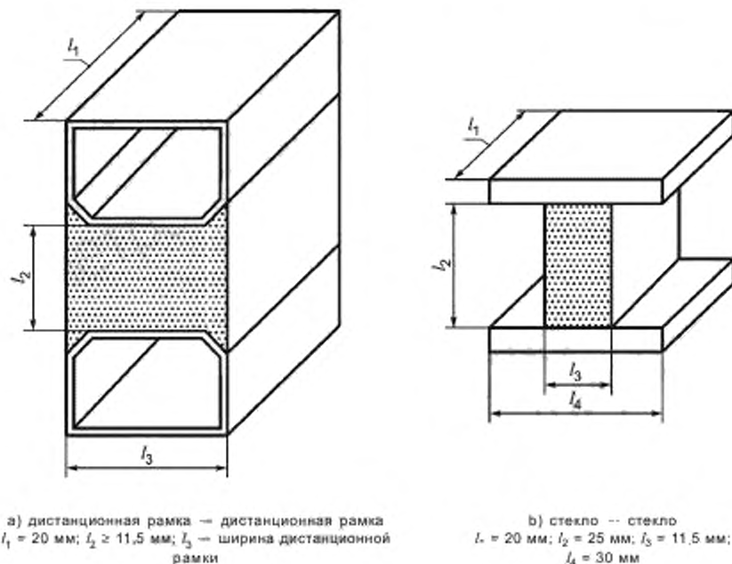
Рисунок F.2 — Образцы для испытаний
