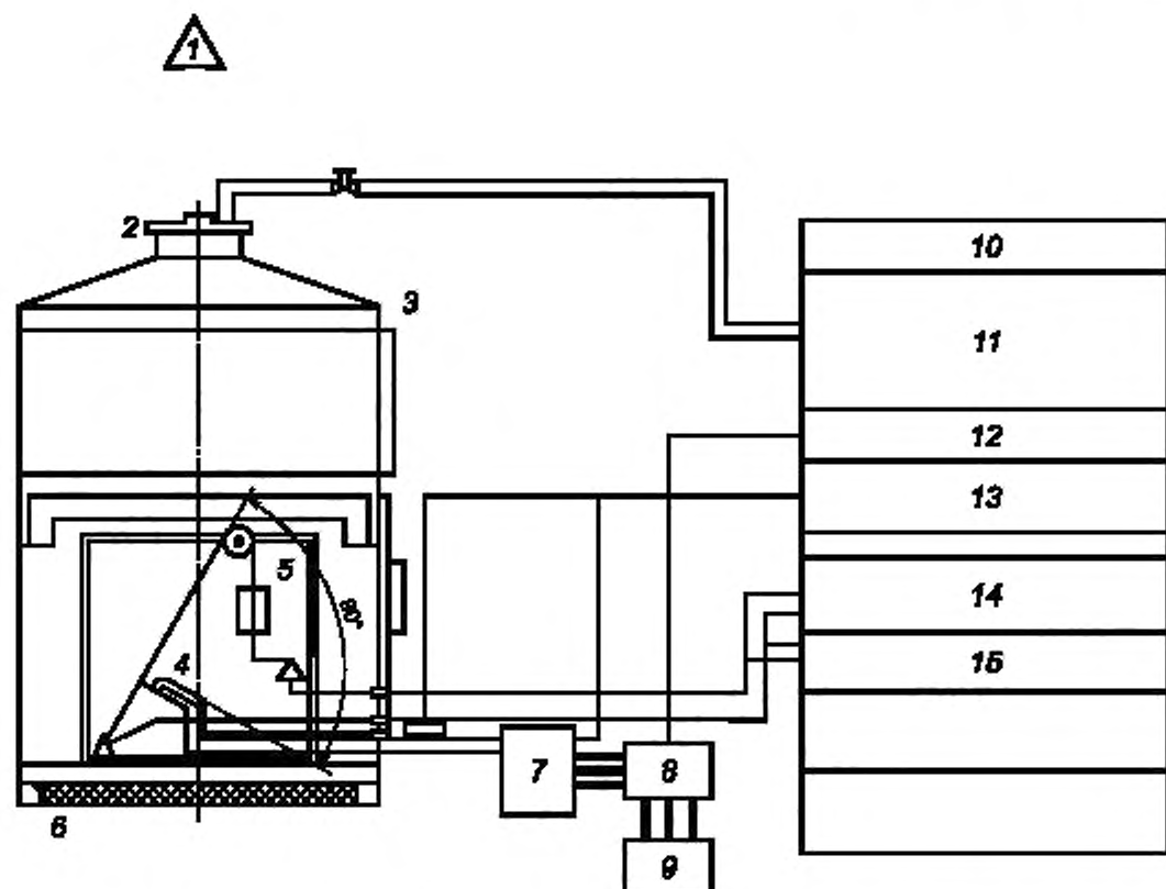
1 — устройство для вентиляции; 2 — верхнее соединительное устройство; 3 — испытательная камера; 4 — горелка Бунзена; 5 — монтаж образца и горелки; 6 — распределительная единица; 7 — электромагнитные клапаны; 8 — контроллер потока массы (см. также позицию 12); 9 — подача газа; 10 — контрольная панель; 11 — анализатор кислорода; 12 — источник питания и устройство индикации (см. также позицию 8); 13 — таймер; 14 — источник питания; 15 — измерение силы тока и напряжения
