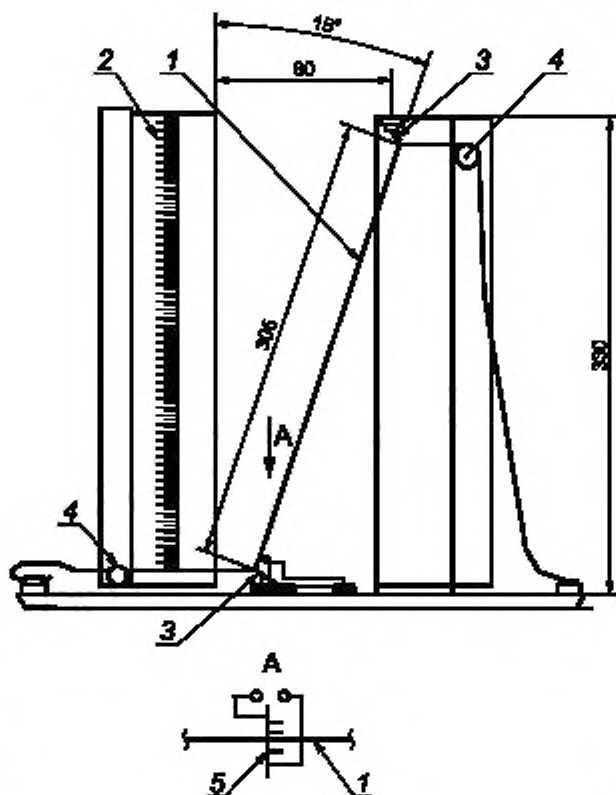
Рисунок 1 — Стандартный держатель образца и установка образца
