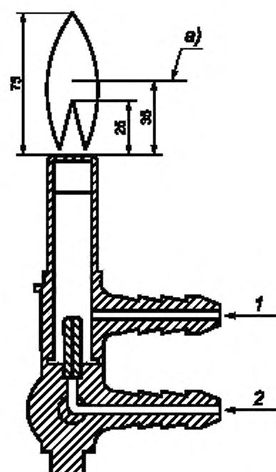
1 — входной воздушный патрубок; 2 — входной клапан для пропана
