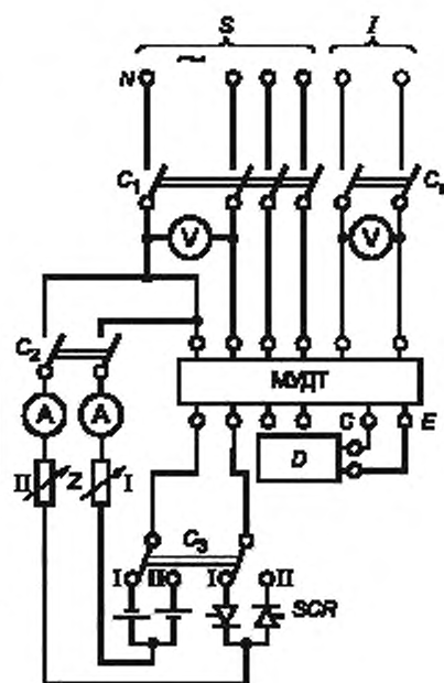
МУДТ выводного типа
