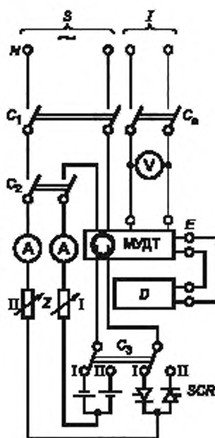
МУДТ со встроенным датчиком
