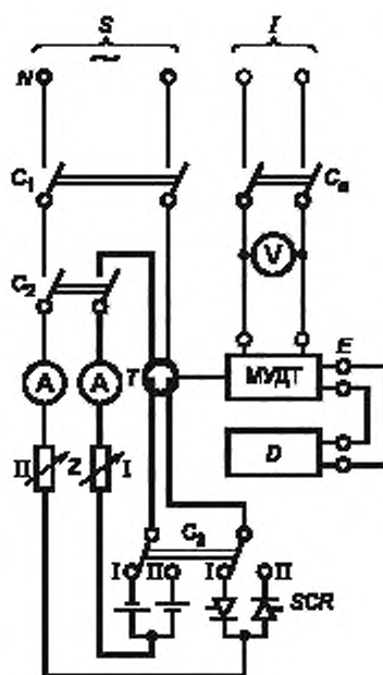
МУДТ с отдельным датчиком
