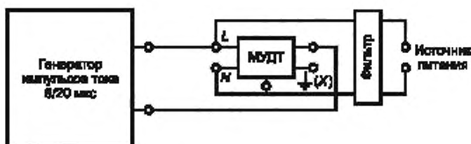
в) МУДТ выводного типа
