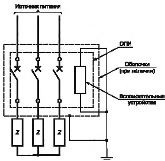
Рисунок F.4 — Испытательная цепь для проверки устойчивости к низкочастотным электромагнитным помехам и испытаний на помехоэмиссию по F.4.1.3, F.4.2, F.4.3, F.4.6, F.4.7.1, F.5.4 и F.6.2 для трехфазного соединения
