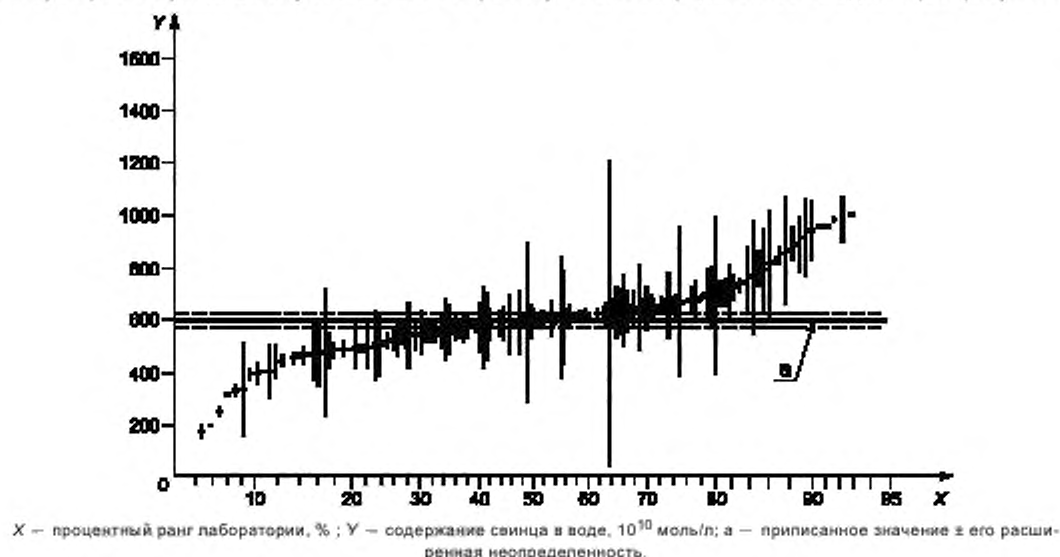
Рисунок 7 — График нормальной функции вероятности с расширенной неопределенностью по данным содержания свинца в воде 156 лабораторий
