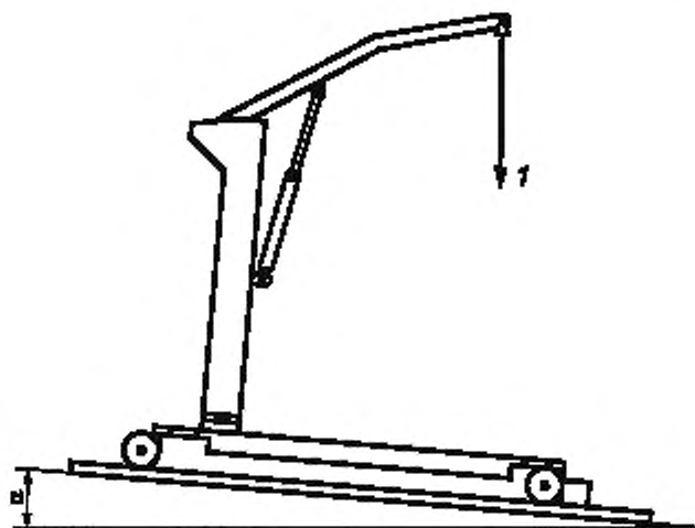
F — испытательная нагрузка, \alpha — угол устойчивости
