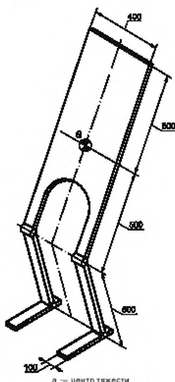
Рисунок 2 — Испытательный макет для поддерживающих и/или приподнимающих подъемников
