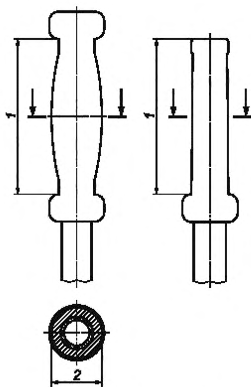
Рисунок 5 — Элементы рукоятки
