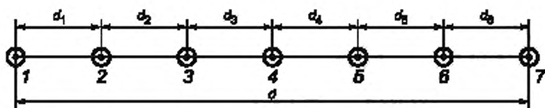
Рисунок 3 — Конфигурация образцовой линии для полной методики испытаний
