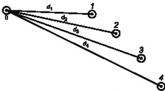
Рисунок 1 — Конфигурация испытательного поля для упрощенной методики испытания
